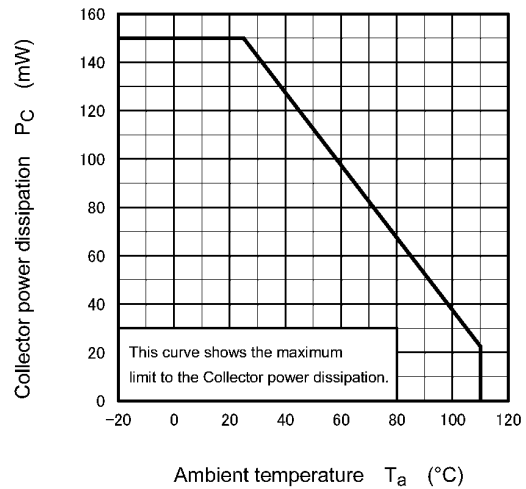
Fig. 11.2 P_C - T_a
