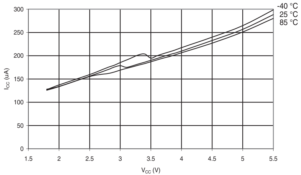
Figure 30-134. ATmega88A: ADC Current vs. V CC (AREF = AV CC )
