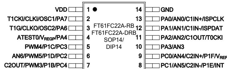
图 1-6 SOP14 / DIP14
