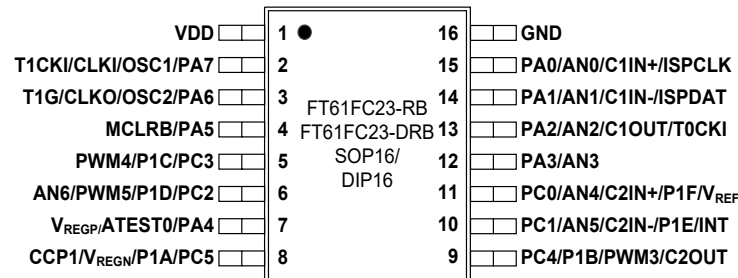
图 1-7 SOP16 / DIP16
