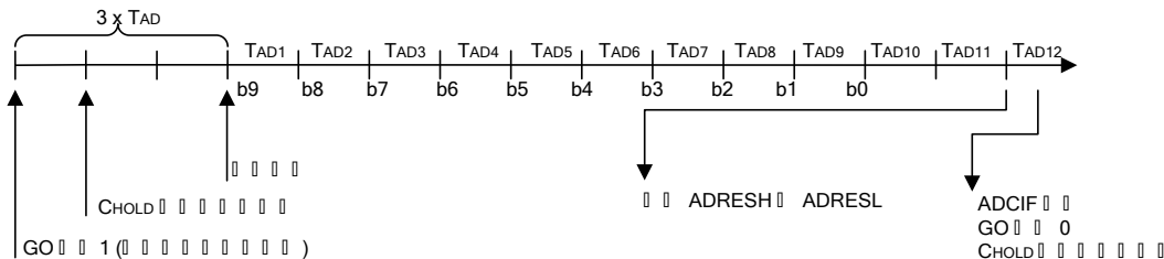
图 12-4 模数转换 T_{AD} 周期
