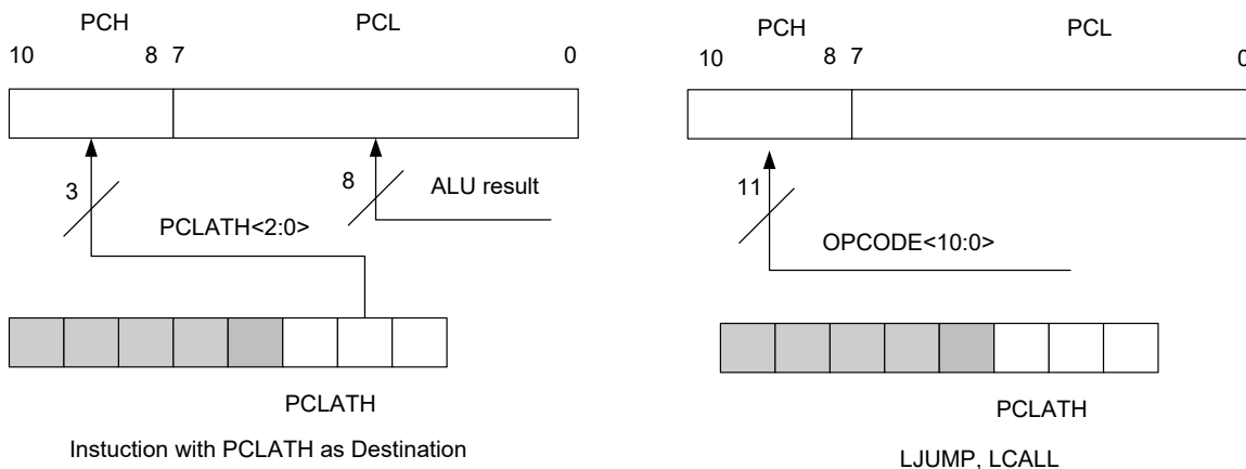
图 17-3 装载 PC 值的不同情况
