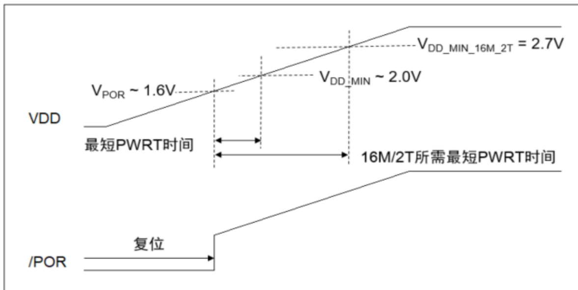
图 3-2 上电过程所需最小 PWRT 时间
