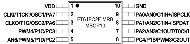
图 1-5 MSOP10
