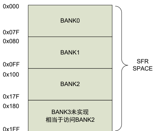
图 17-2 间接寻址
