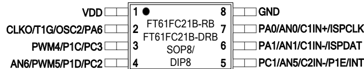
图 1-4 SOP8 / DIP8 (B)
