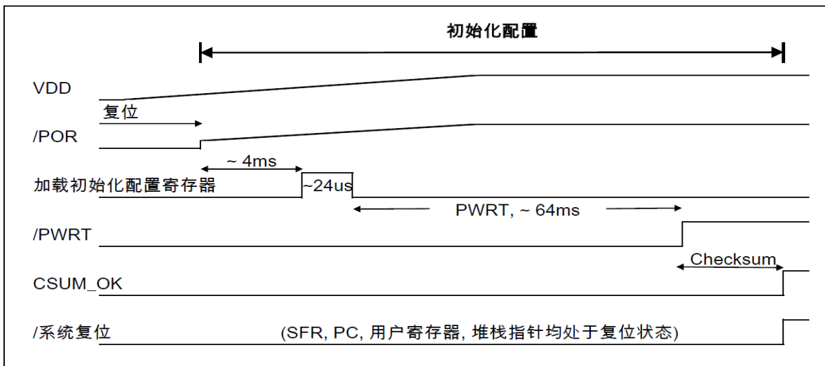
图 3-1 上电时序 (PWRT 和 Checksum 使能)
