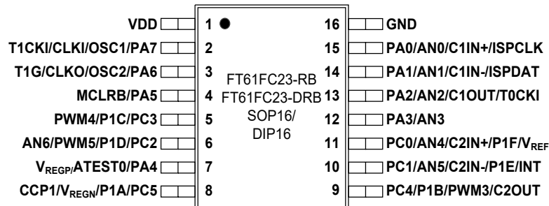
图 1-7 SOP16 / DIP16
